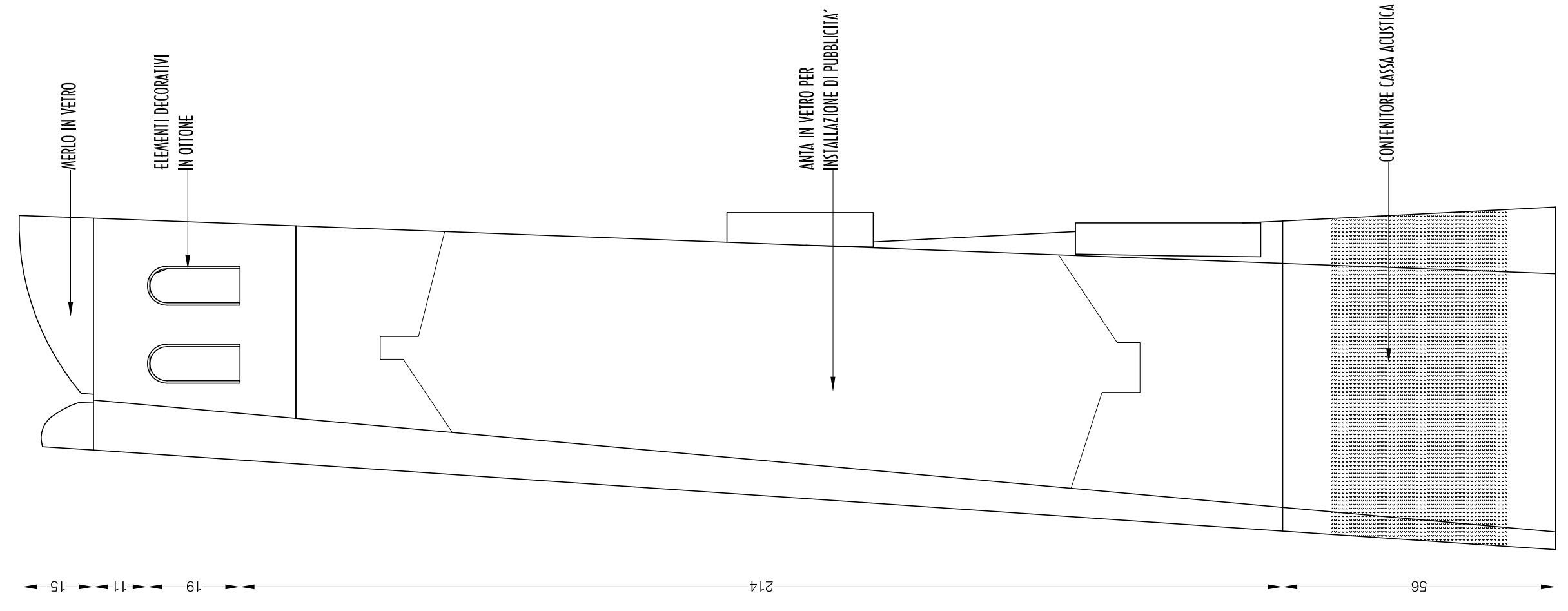
PROSPETTO "D"
