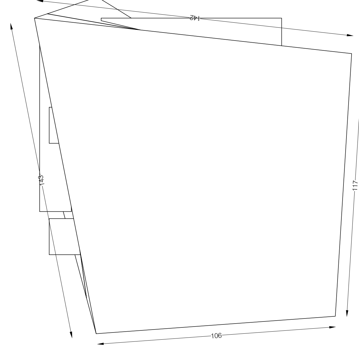
PIANTA INFERIORE
